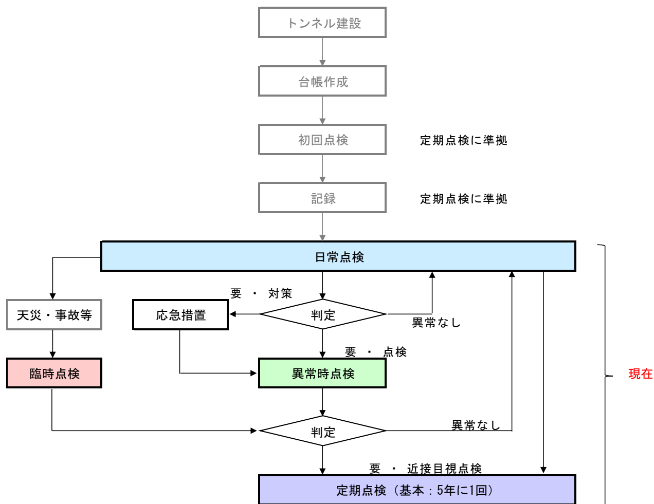
図 3-1 点検の基本フロー（建設～定期点検）
