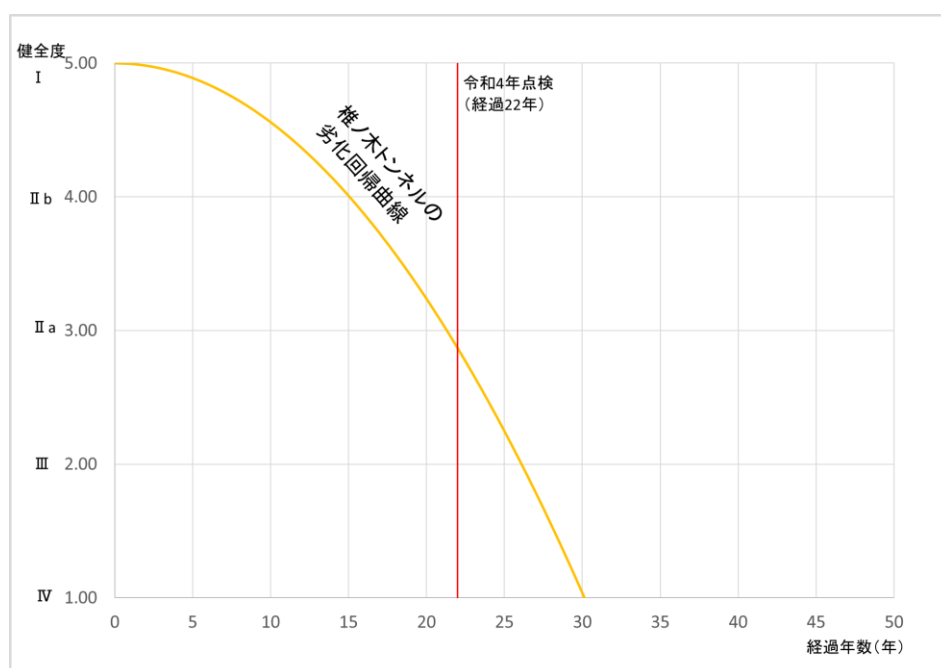
図 5-2 椎ノ木トンネルにおける劣化予測の回帰分析図
