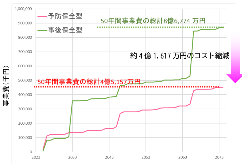
図 6-2 トンネルの維持管理予算の推移
