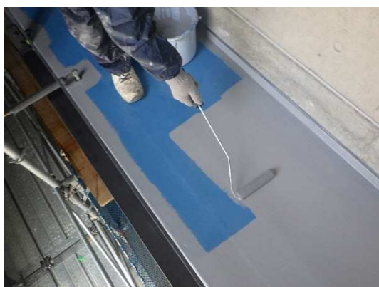
外部バルコニー部塗膜防水(仕上げ)
