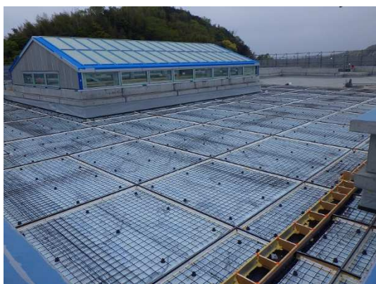
屋上 西面 メッシュ敷き状況
