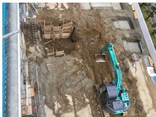
東面 外構工事(熱源装置・オイルタンク)
