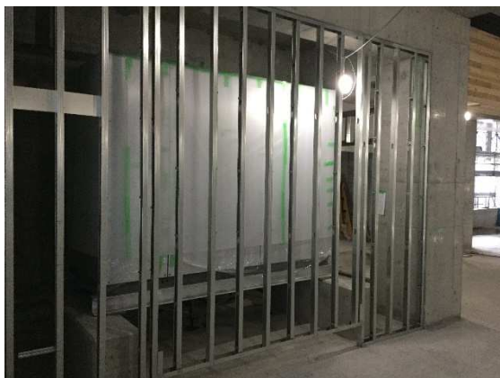
間仕切壁(下地) 組立状況
