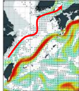
東シナ海海域の海流図 (気象庁 HPより)
